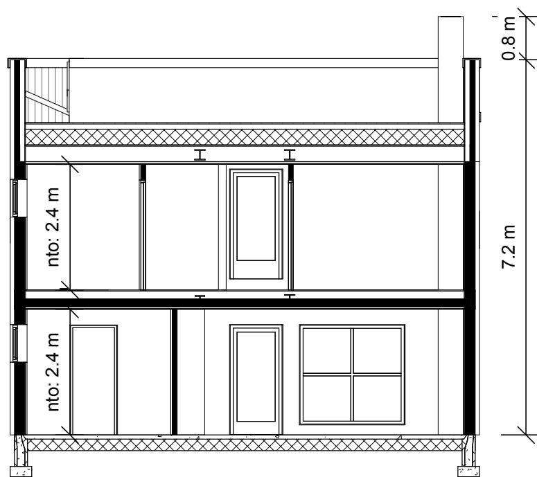
SNITT A-A
